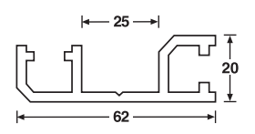
6165 AL racková lišta dvojité s drážkou
