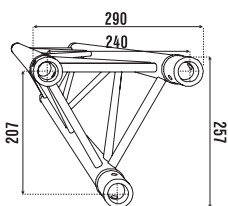
B: trubky: 50x2mm výplet: 16x2mm
