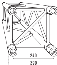
B: trubky: 50x2mm výplet: 16x2mm
