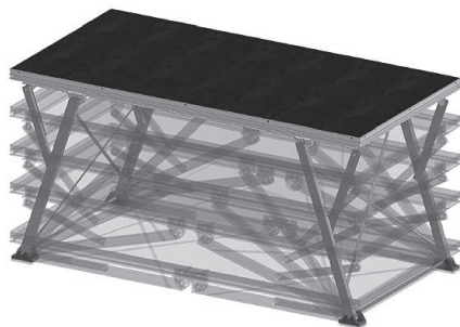
MILOS X-stage S1 200×100 cm, výškově nastavitelný pódiový modul na 20, 40, 60, 80 a 100 cm, ALU rám + překližka 22 mm, max. zátěž 750 kg/m 2 , hmotnost 58 kg, bez spojovacích konektorů
