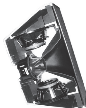
AX364 pohľad na vnútorné usporiadání
